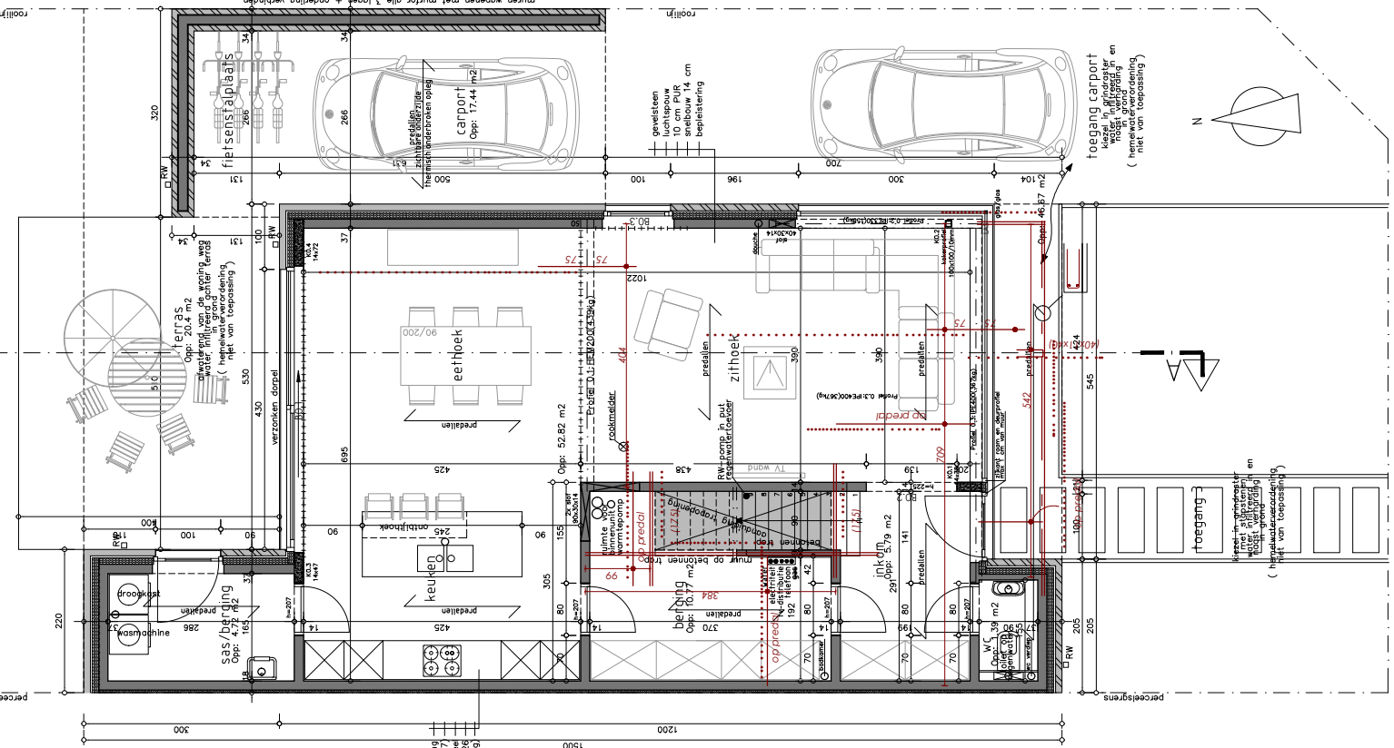
Gelijkvloers Lot 27 Opp: 90.93 m 2 woning + 20.28 m 2 carport
